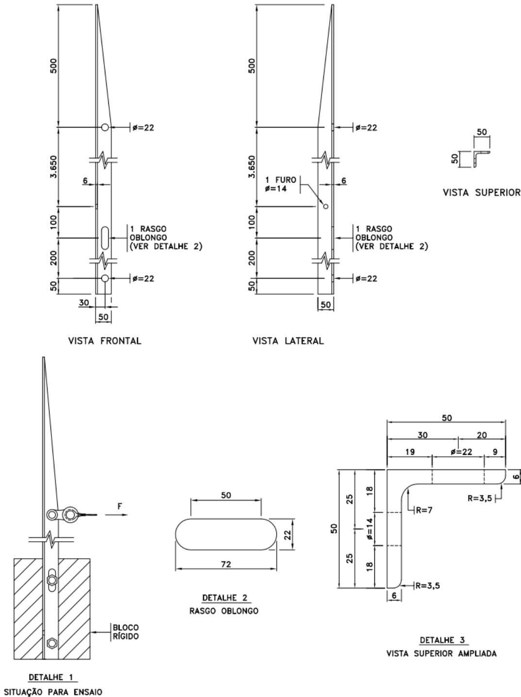
Figura 1 – Desenho de haste para para-raios “L”
